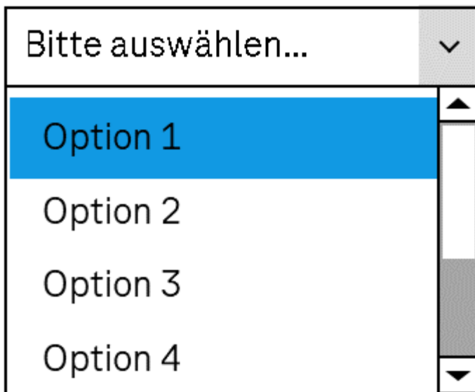
Abbildung: Ausklappliste
