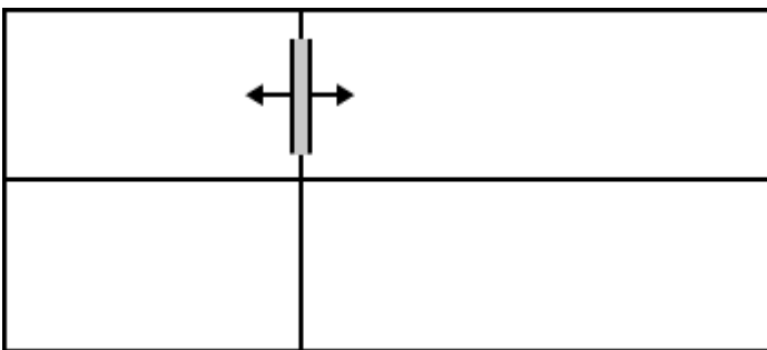
Abbildung: Bereichstrenner
