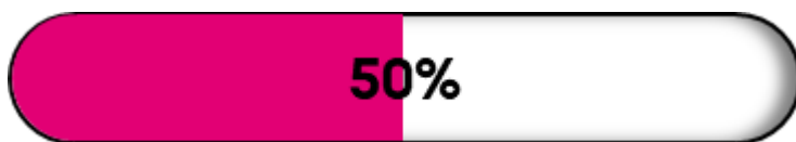
Abbildung: Fortschrittsanzeige
