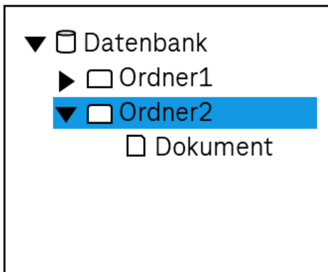
Abbildung: Baumstruktur
