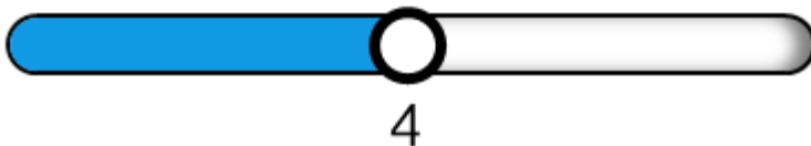
Abbildung: Schieberegler
