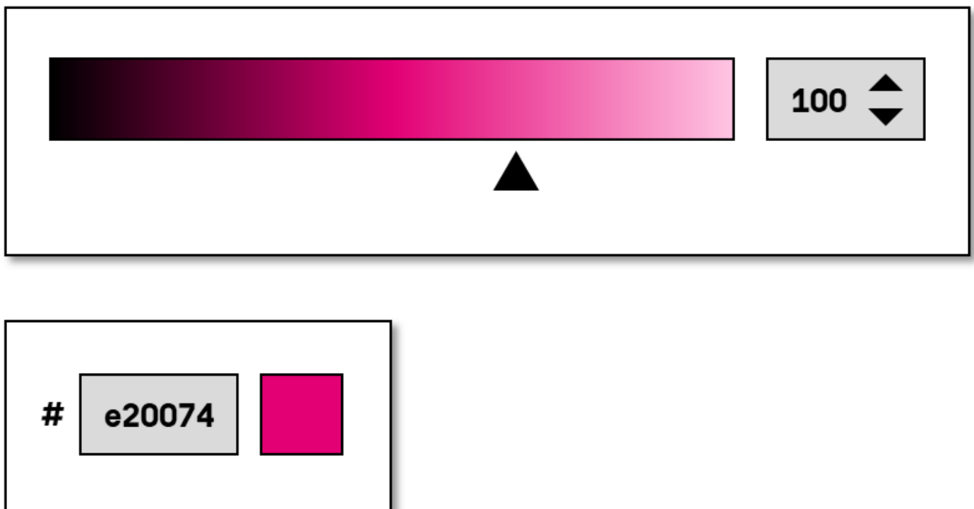
Abbildung: Farbwähler
