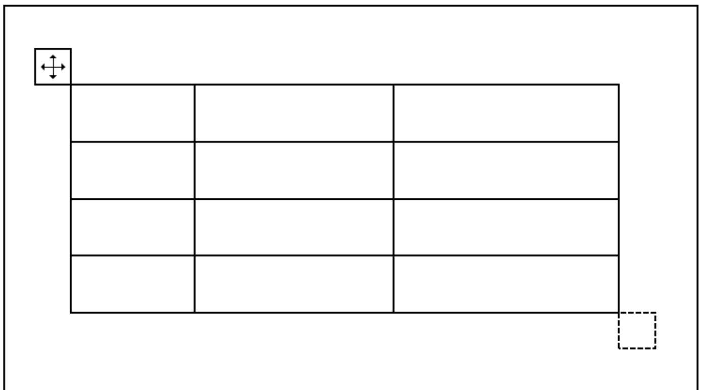
Abbildung: Griff
