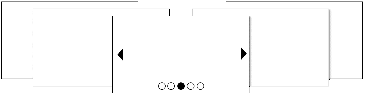
Abbildung: Karussell
