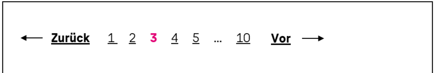
Abbildung: Paginierung
